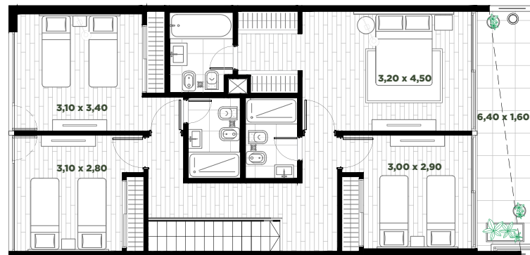
1 PISO
